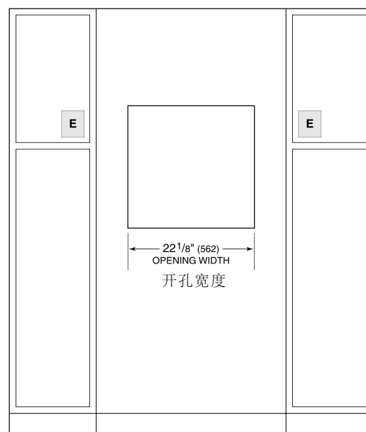
FRONT VIEW 前视图
