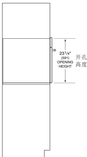
SIDE VIEW 側视图
